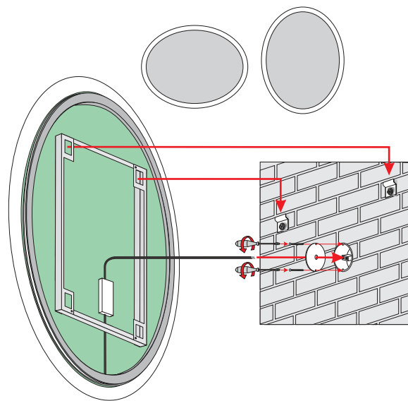
Installation position Montageposition/ Pozycja montażu
